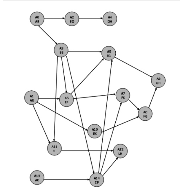
شکل ۵: گراف وابستگی مخزن قانون جدول ۲
