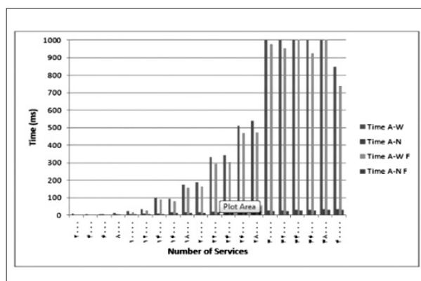
شکل ۱۲: نمودار مقایسه زمان اجرا در بازه‌های A\_W و A\_N با ورودی-خروجی B\_M (دو روش CAUT-K و Brahmi)
