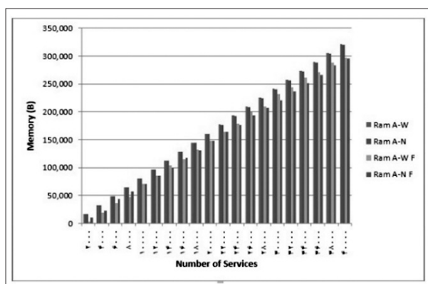
شکل ۱۳: نمودار مقایسه مصرف حافظه در بازه‌های A\_W و A\_N با ورودی-خروجی B\_M (دو روش CAUT-K و Brahmi)
