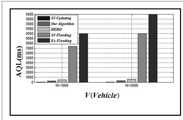
نمودار ۷: بررسی تأثیر تعداد وسایل نقلیه، V ، بر میانگین تأخیر در هر درخواست
